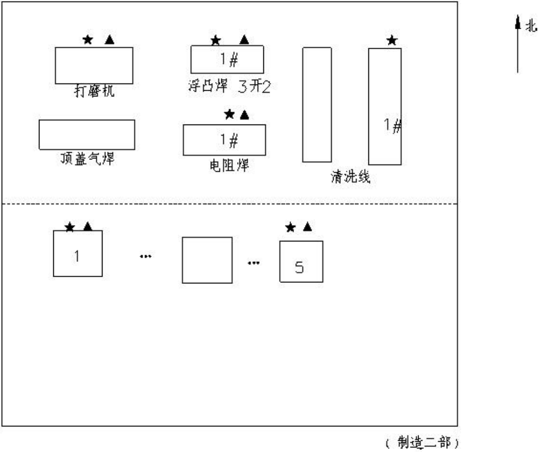
现场布点示意图
