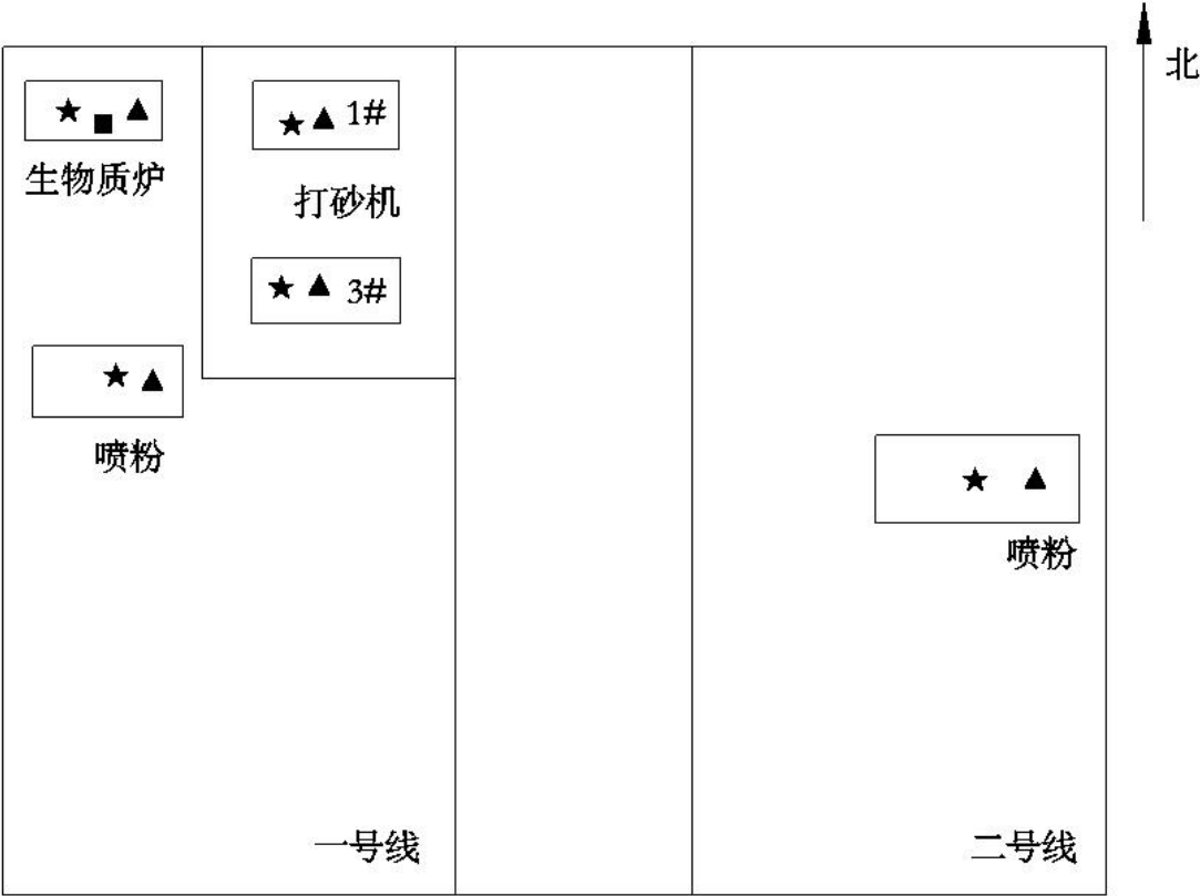
现场布点示意图
